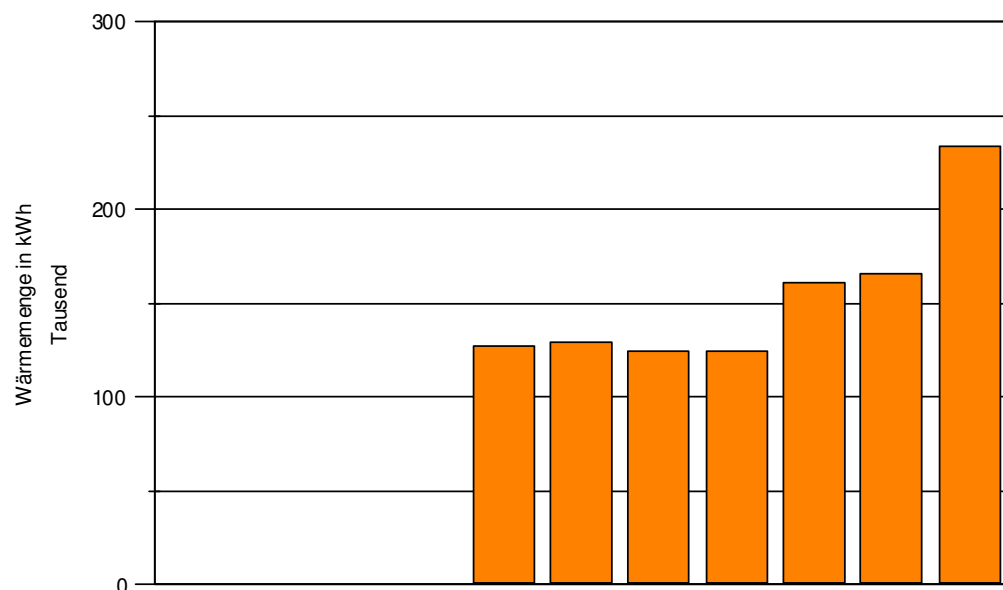
Waldorfschule Weimar · Heizenergieverbrauch gesamt
